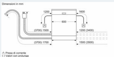
Dimensioni in mm Presa di corrente Valori con prolunga
