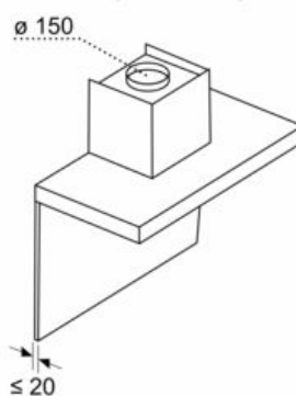
Dimensioni in mm Profondità dal pannello a parete
