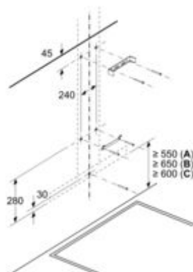
Dimensioni in mm Profondità dal pannello a parete
