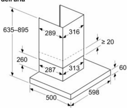
Dimensioni in mm Apparecchio in modalità di estrazione dell'aria
