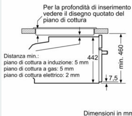
Montaggio con un piano di cottura.
