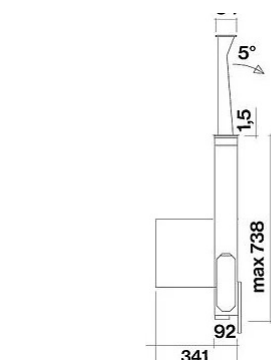
Vista laterale installazione con motore posteriore
