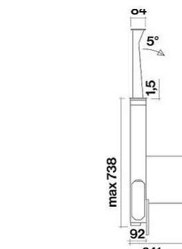
Vista laterale installazione con motore anteriore
