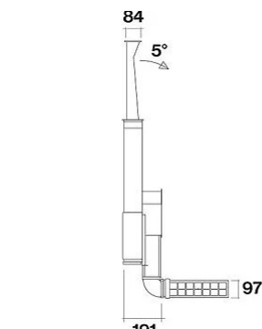
Vista laterale installazione con motore slim anteriore
