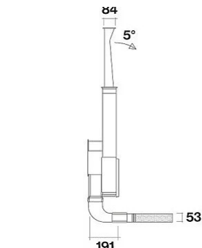
Vista laterale installazione con motore slim posteriore, filtro sottobase KACL.951 (h 60mm)
