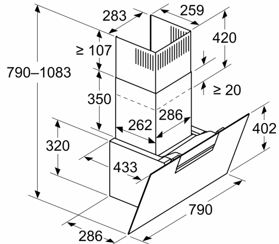
Dimensioni in mm Apparecchio in modalità di ricircolo d'aria
