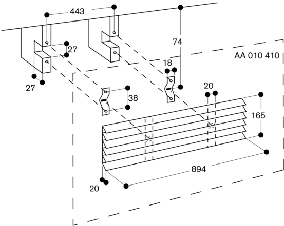
AA 010 410 griglia di uscita aria
