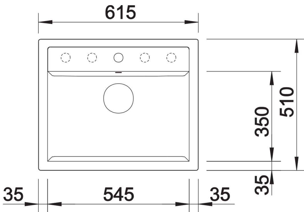
Vista superiore
