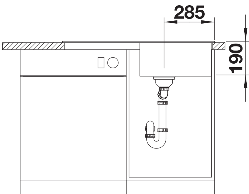
Vista frontale
