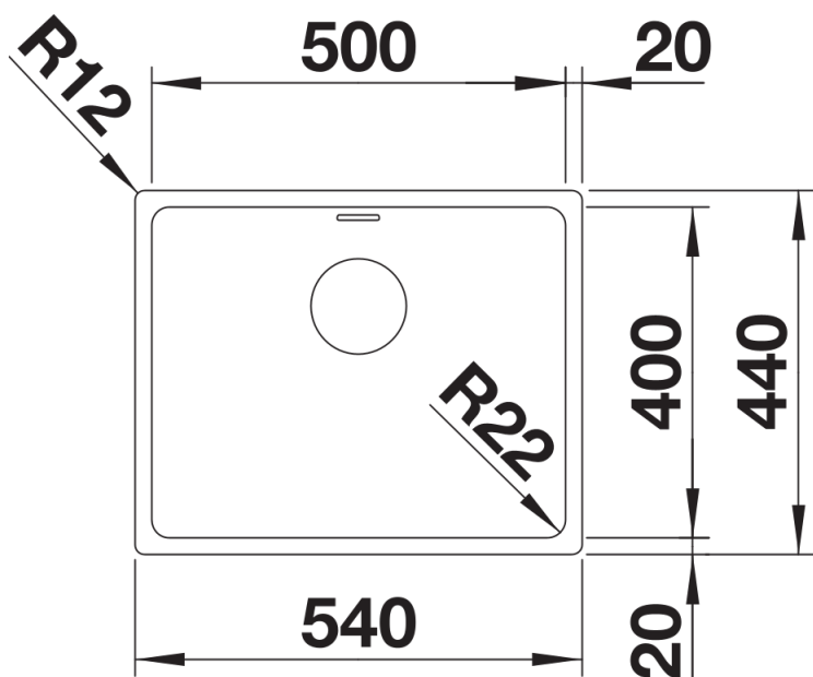
Vista superiore
