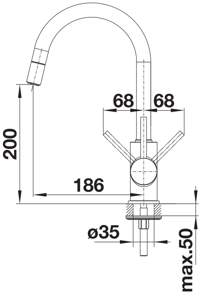
Vista laterale
