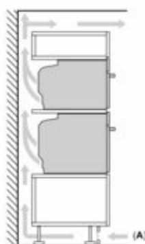
Montaggio di due apparecchi sovrapposti Ricambio dell'aria
